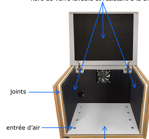
laine de roche compressé recouvertes de fibre de verre lavable et résistant à la chaleur
